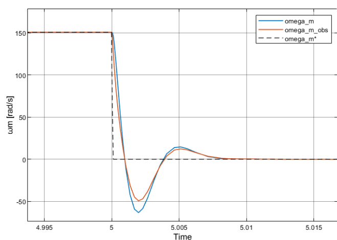
Figura 44: Detalle en t = 5s
