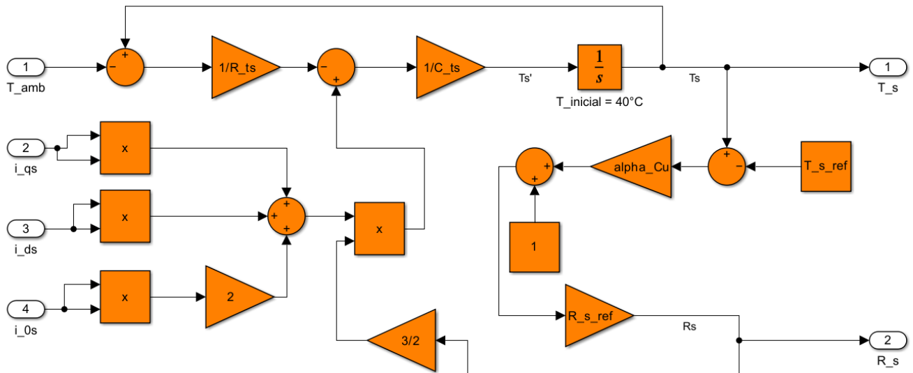
Figura 5: Subsistema térmico
