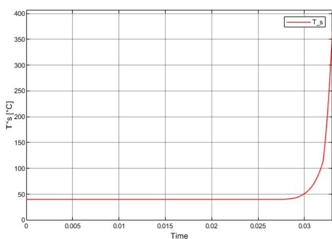
Figura 70: Curva de temperatura con \tau = 20 \text{ s}
